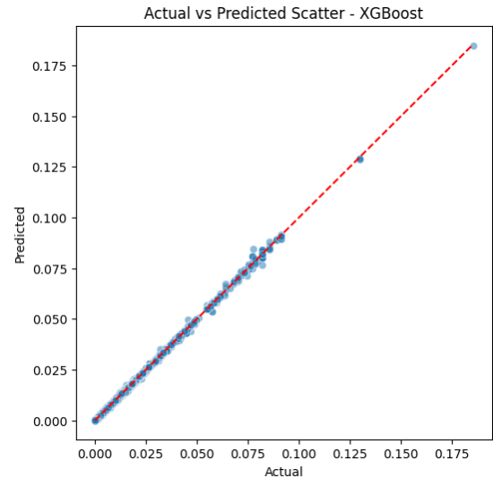
Fig. 13 Actual vs Predicted Scatter Plot-XGBoost
