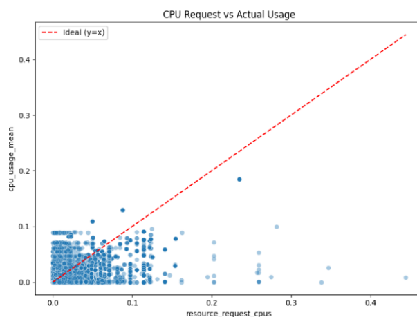
Fig. 6 CPU Request vs Actual Usage
